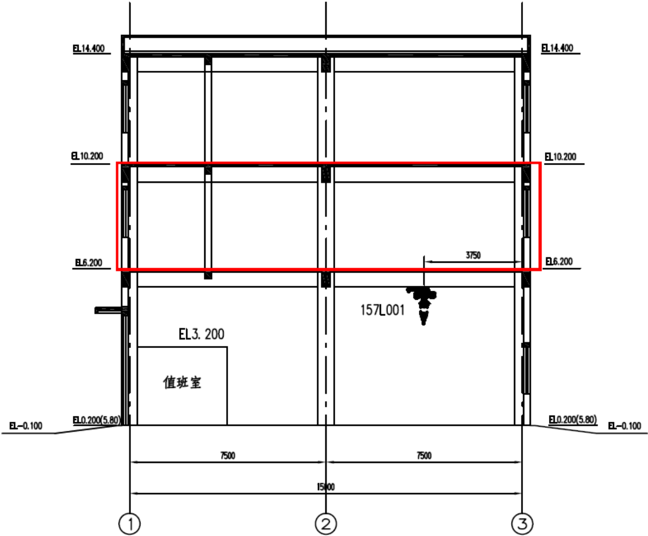
A-A剖视
